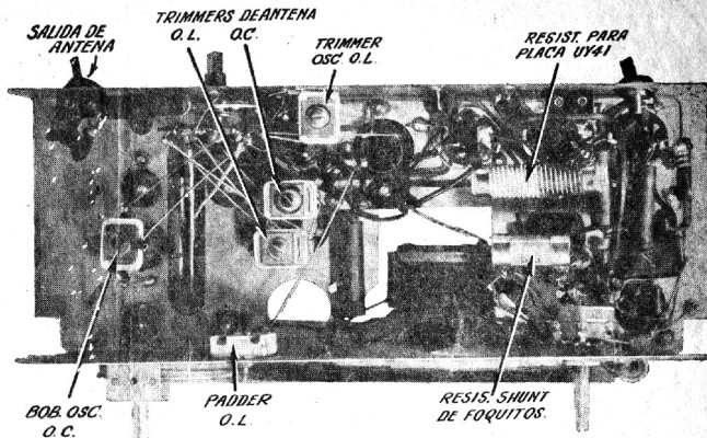
VISTA INFERIOR DEL CHASIS
