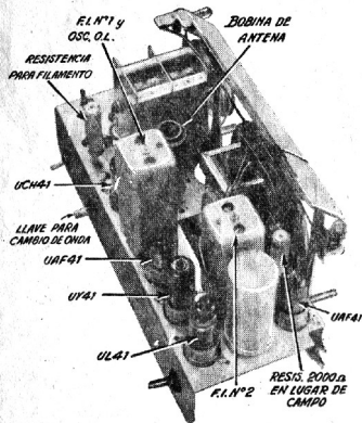
VISTA SUPERIOR DEL CHASIS
